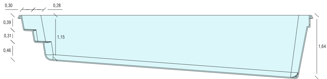
CORTE C-C
