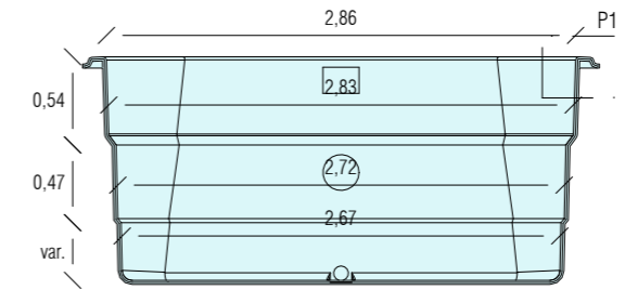
CORTE B-B
