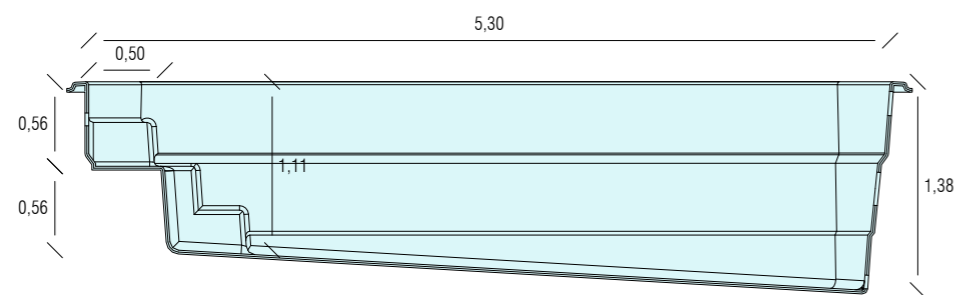
CORTE C-C
