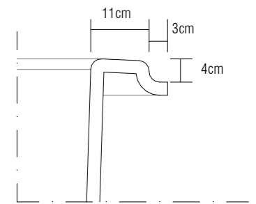
PORMENOR P1 - ESC 1:10
