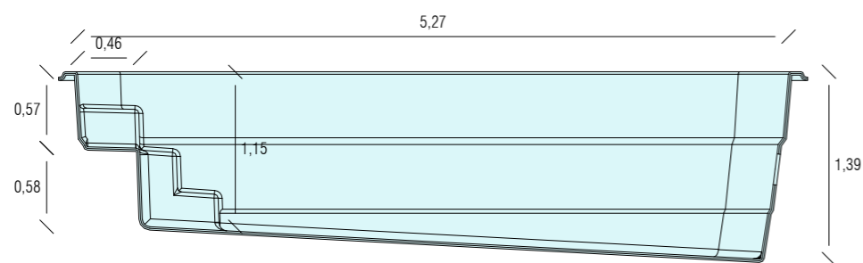
CORTE C-C
