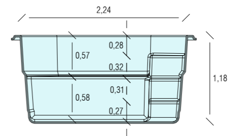
CORTE A-A
