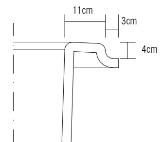
PORMENOR P1 - ESC 1:10
