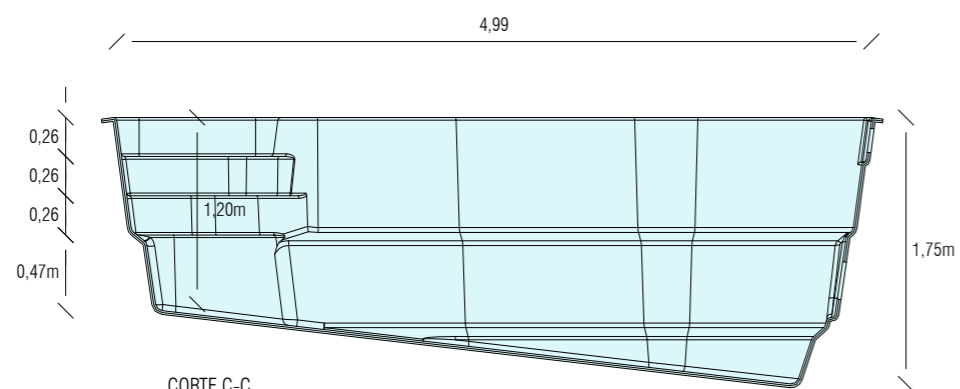
CORTE C-C
