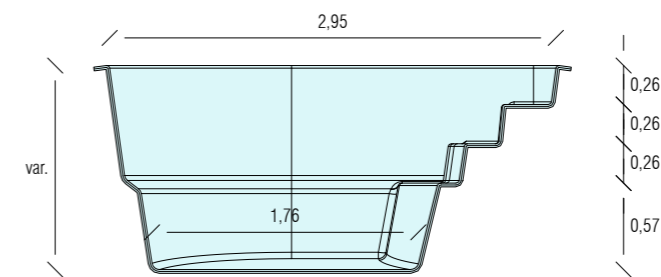
CORTE A-A
